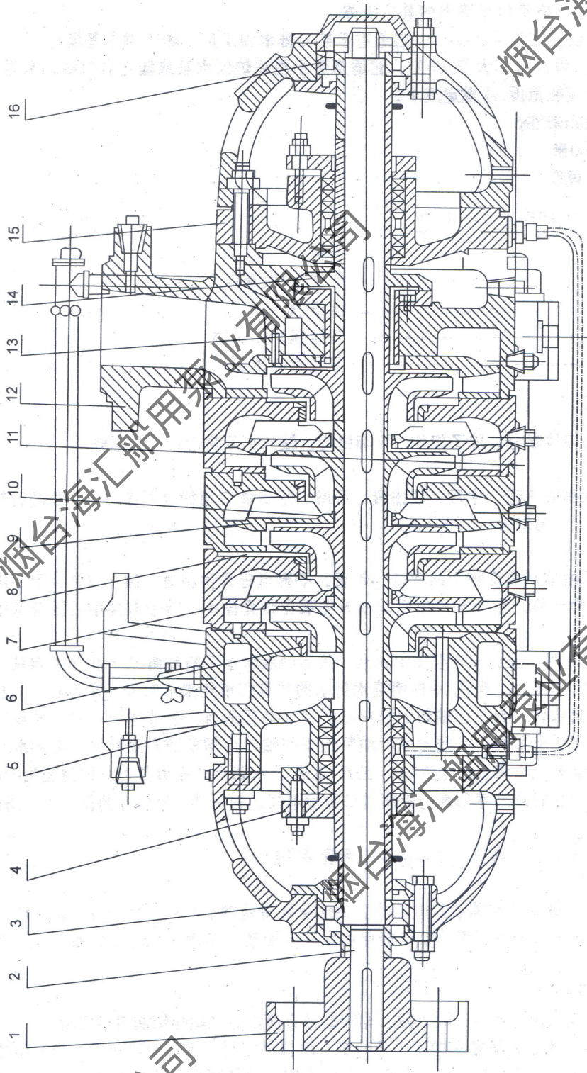
图1 D型泵结构图
