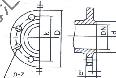
法兰图 Flange Drawing
