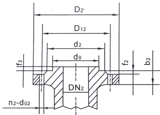
吐出口法兰
